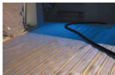
Berechnung Kabelabstand: m^2 : Kabellänge = Kabelabstand z.B. 20 m^2 : 110 lm = 18,2 cm Abstand
